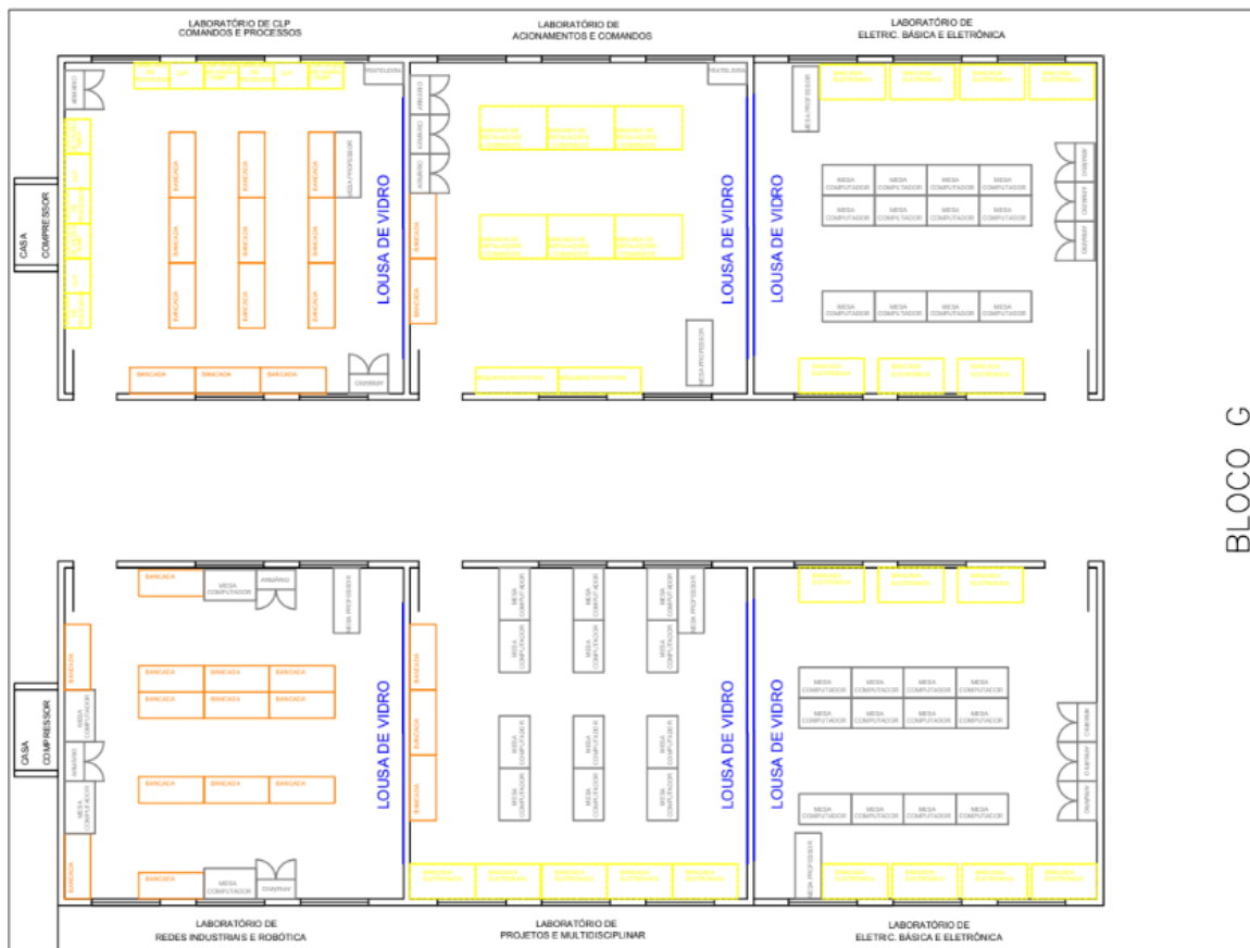
Figura 18.4 Planta baixa de espaço proposto para laboratórios didáticos.
